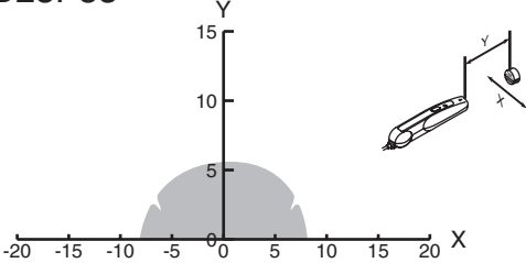
V600-D23P55
