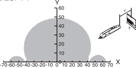
V600-D2KR16
