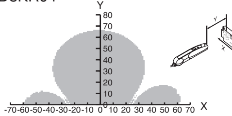
V600-D8KR13
