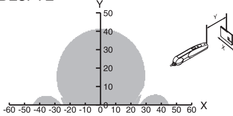
V600-D8KR04
