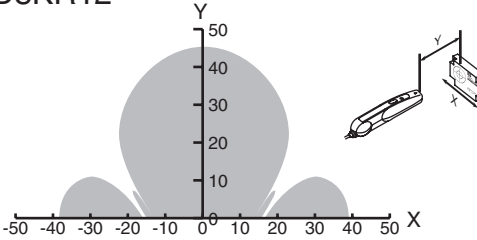
V600-D8KR12
