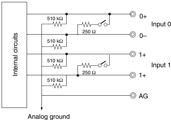
Analog Inputs
